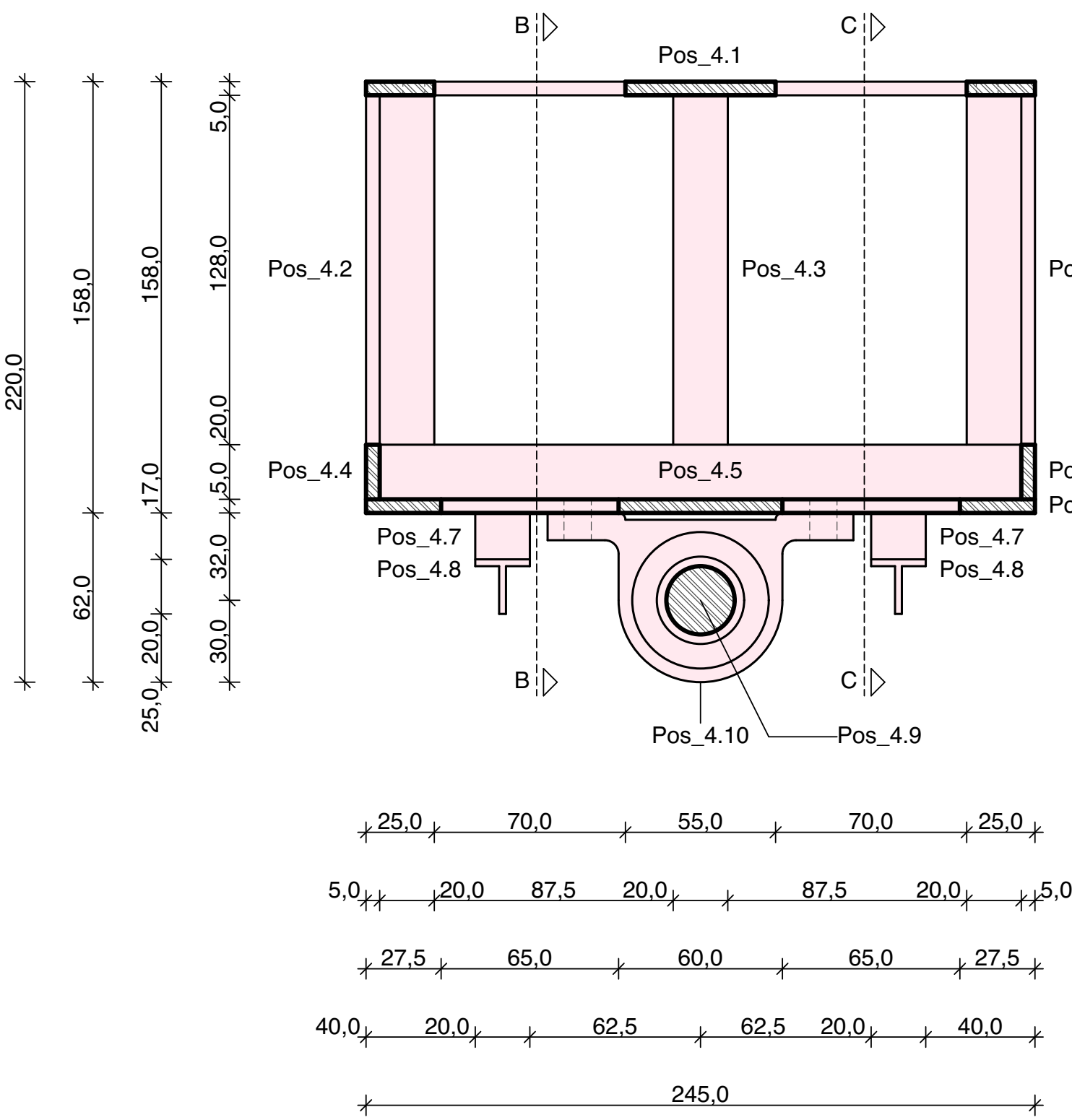
Assembly_Section (A-A)
