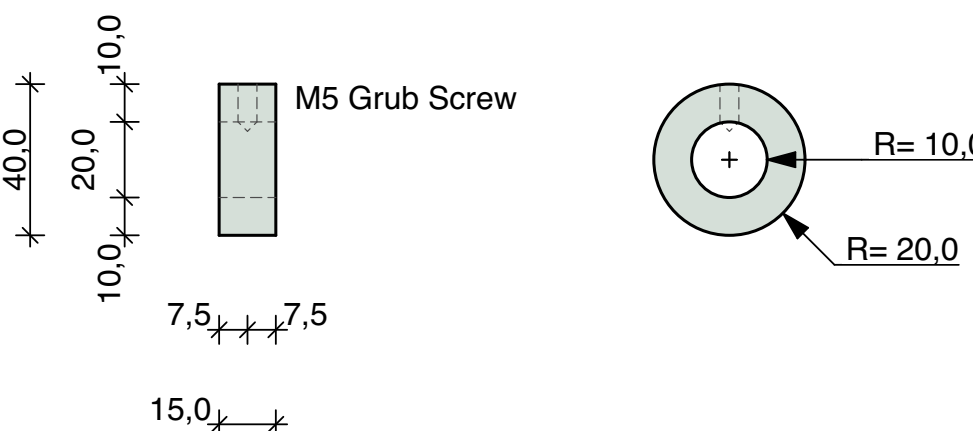
Pos_6.2.7 2 Stück Cuff 20 x 40 x 15 mm
